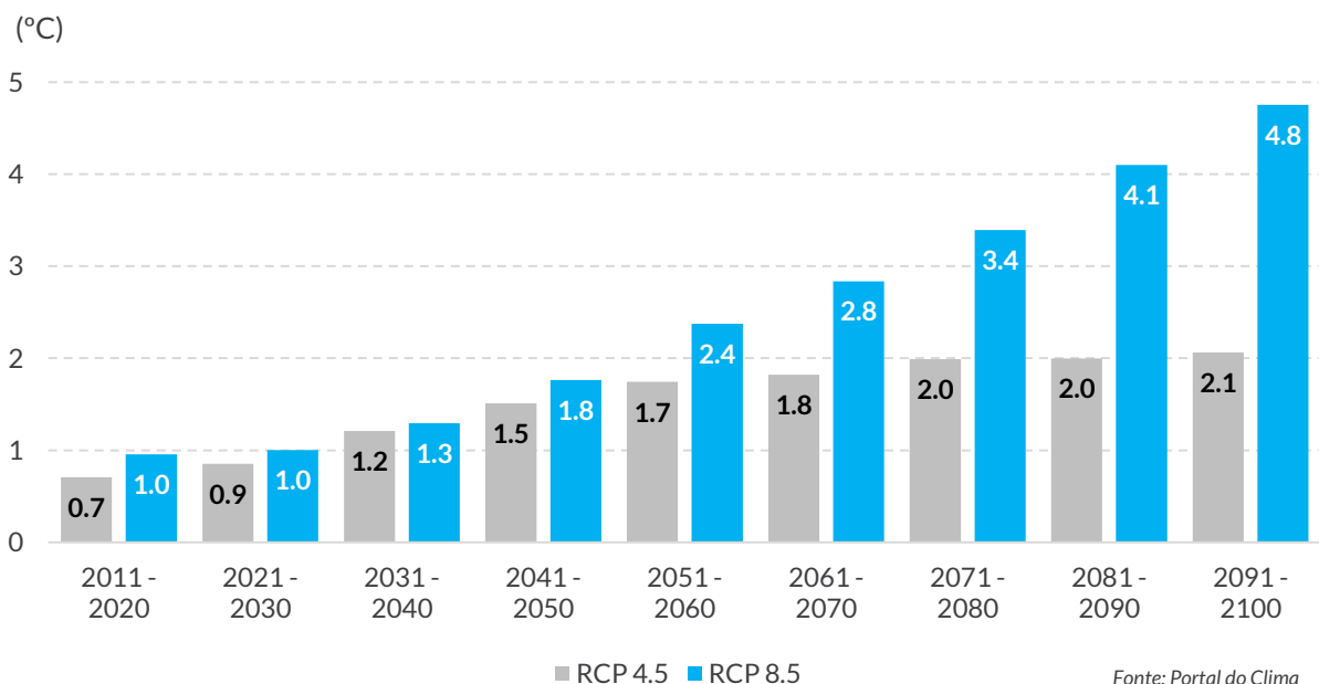
Gráfico 16. Anomalias da temperatura média máxima (°C) na região de Viseu Dão Lafões
