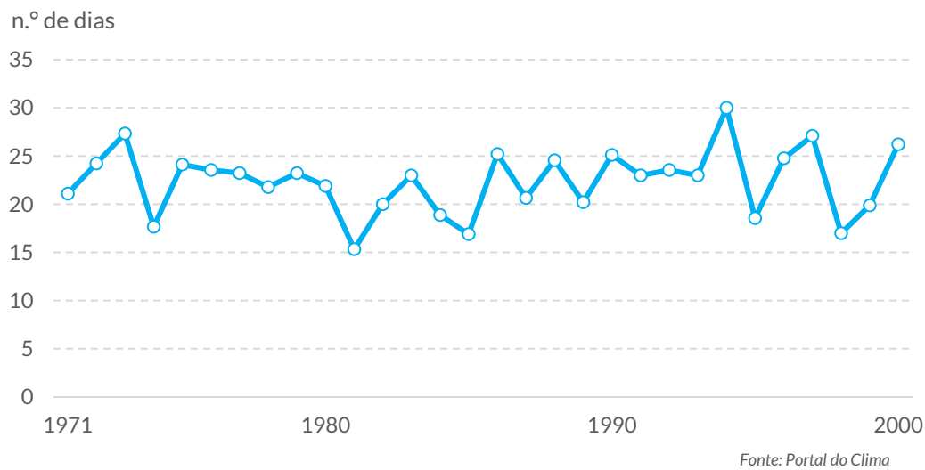
Gráfico 29. Histórico simulado de dias com precipitação superior a 20mm (n.º) na região de Viseu Dão Lafões
