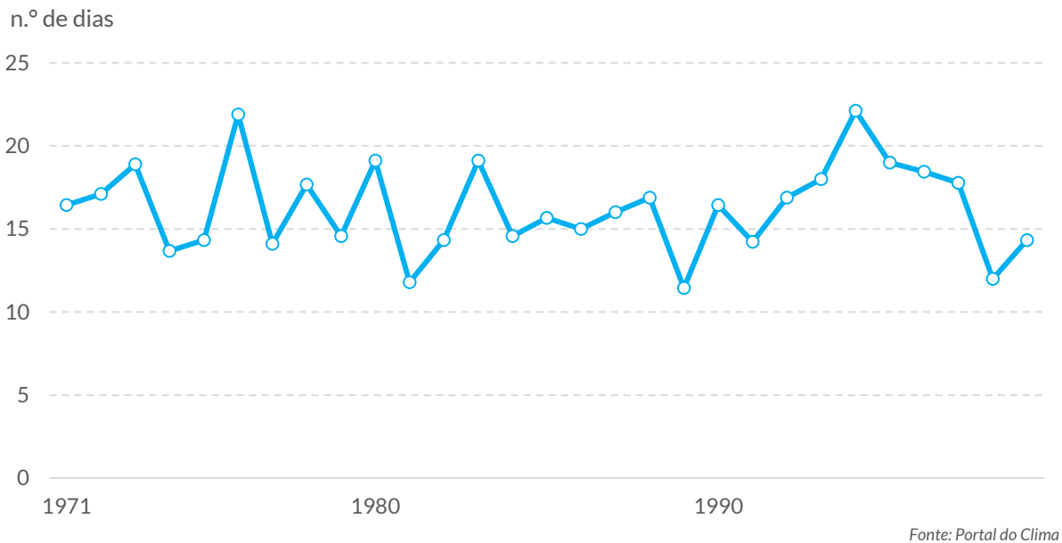
Gráfico 33. Histórico simulado de dias consecutivos com chuva (n.º) na região de Viseu Dão Lafões
