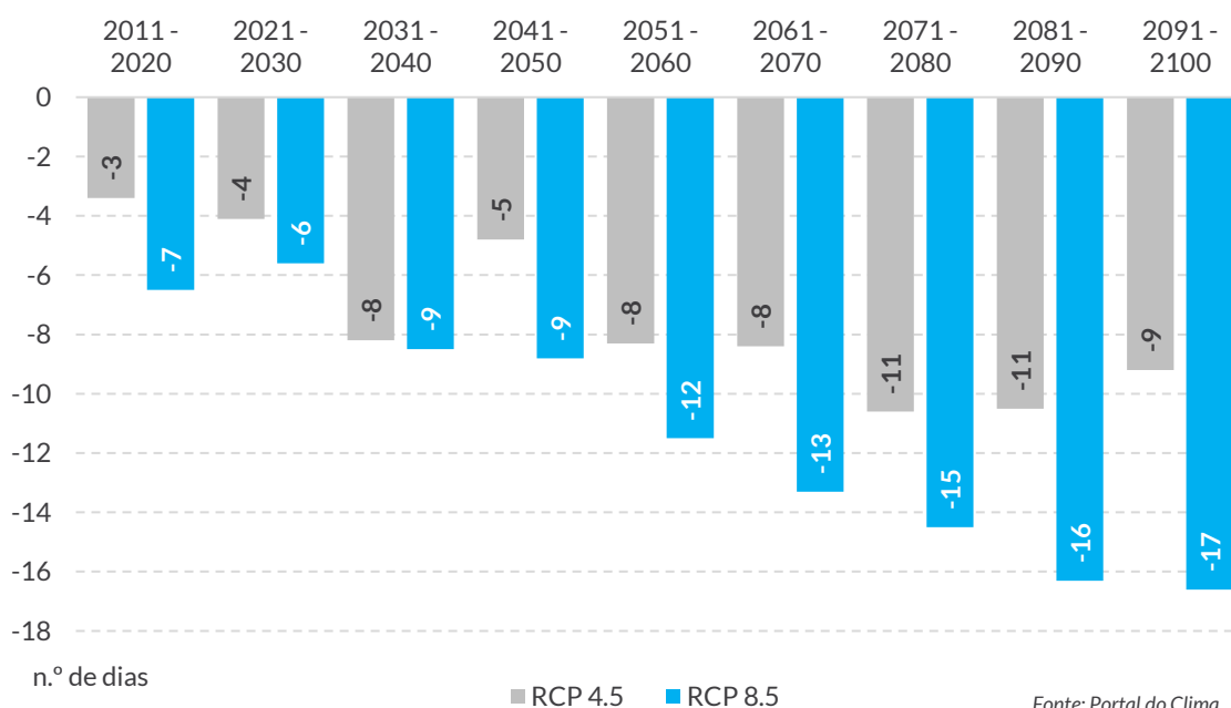
Gráfico 22. Anomalias de dias de geada (n.º) na região de Viseu Dão Lafões
