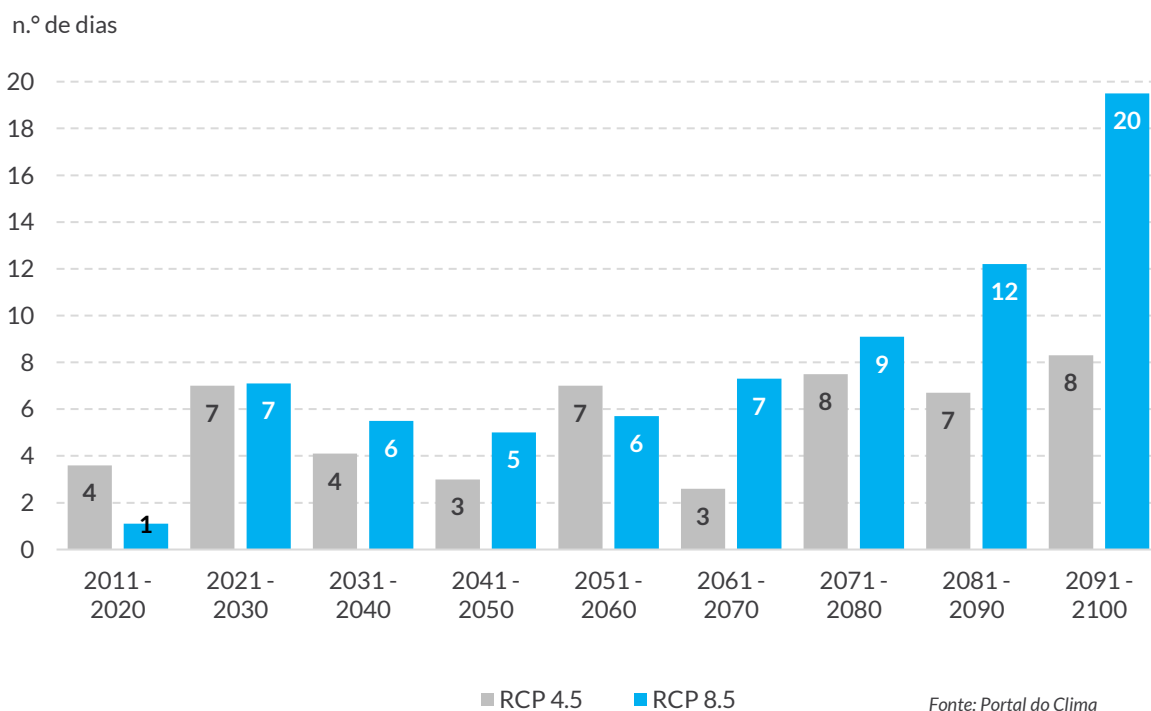
Gráfico 32. Anomalias de dias consecutivos sem chuva (n.º) na região de Viseu Dão Lafões
