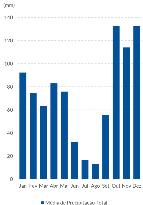
Gráfico 9. Valores de precipitação na Guarda, 1981-2010
