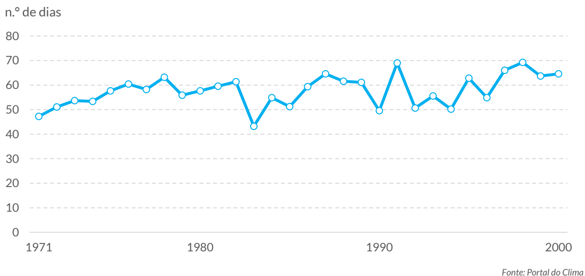
Gráfico 17. Histórico simulado de dias de verão (n.º) na região de Viseu Dão Lafões
