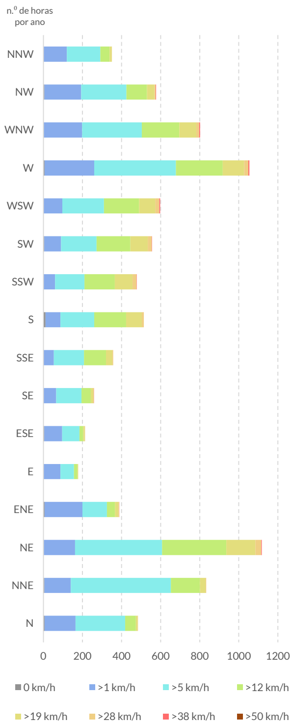
Gráfico 10. Número de horas de vento por ano, velocidade e direção em Aguiar da Beira, média dos últimos 30 anos
