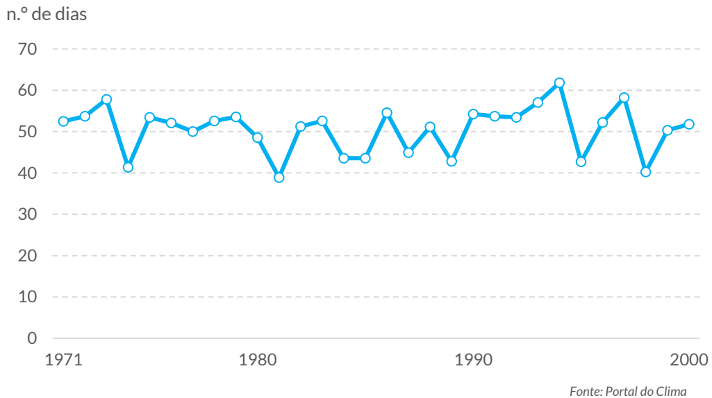
Gráfico 27. Histórico simulado de dias com precipitação superior a 10mm (n.º) na região de Viseu Dão Lafões
