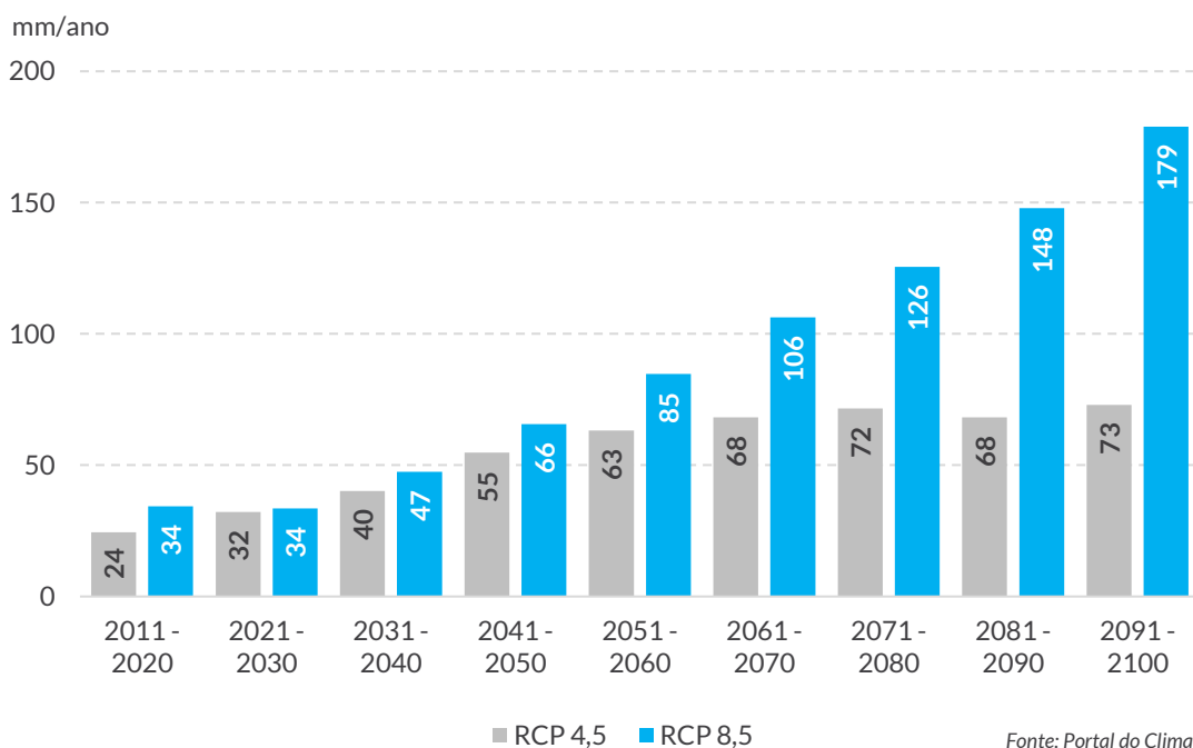
Gráfico 36. Anomalias de evapotranspiração (mm/ano) na região de Viseu Dão Lafões
