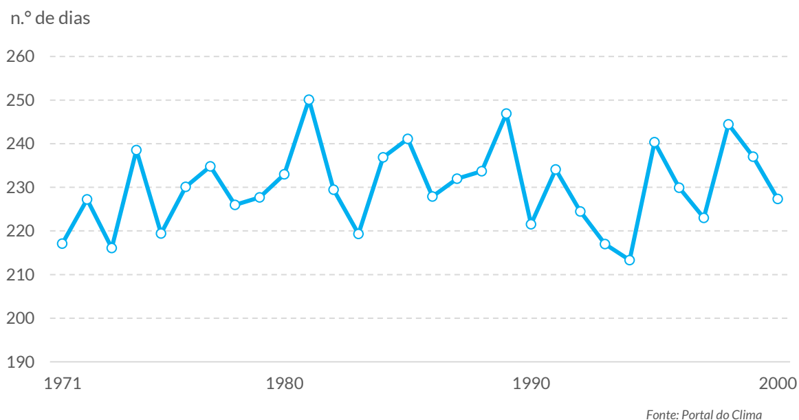
Gráfico 25. Histórico simulado de dias sem chuva (n.º) na região de Viseu Dão Lafões
