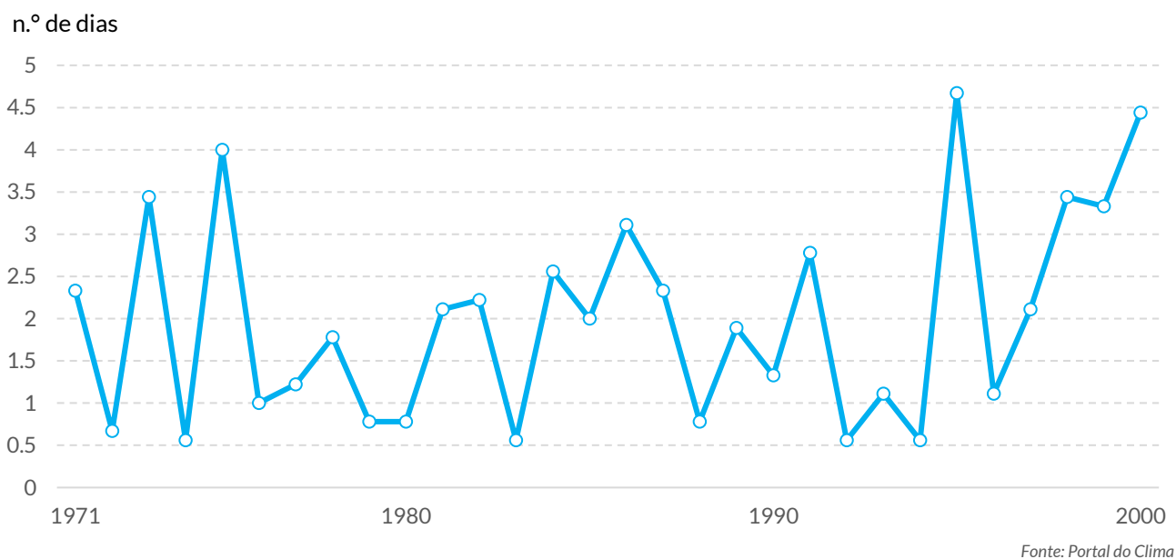
Gráfico 19. Histórico simulado de dias muito quentes (n.º) na região de Viseu Dão Lafões
