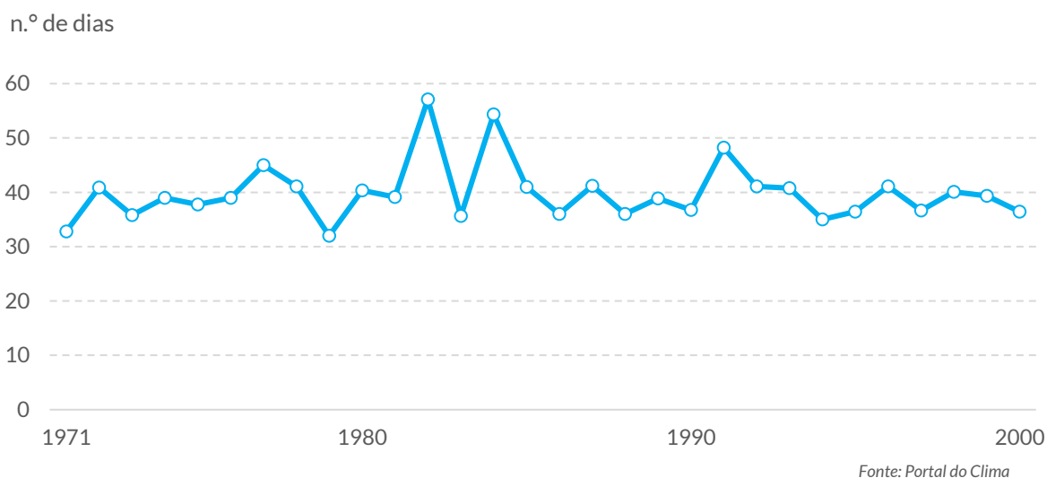
Gráfico 31. Histórico simulado de dias consecutivos sem chuva (n.º) na região de Viseu Dão Lafões
