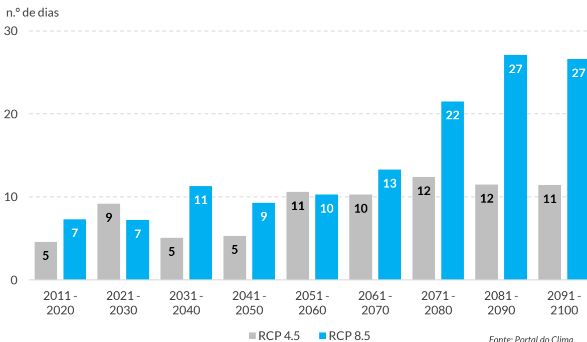
Gráfico 26. Anomalias de dias sem chuva (n.º) na região de Viseu Dão Lafões
