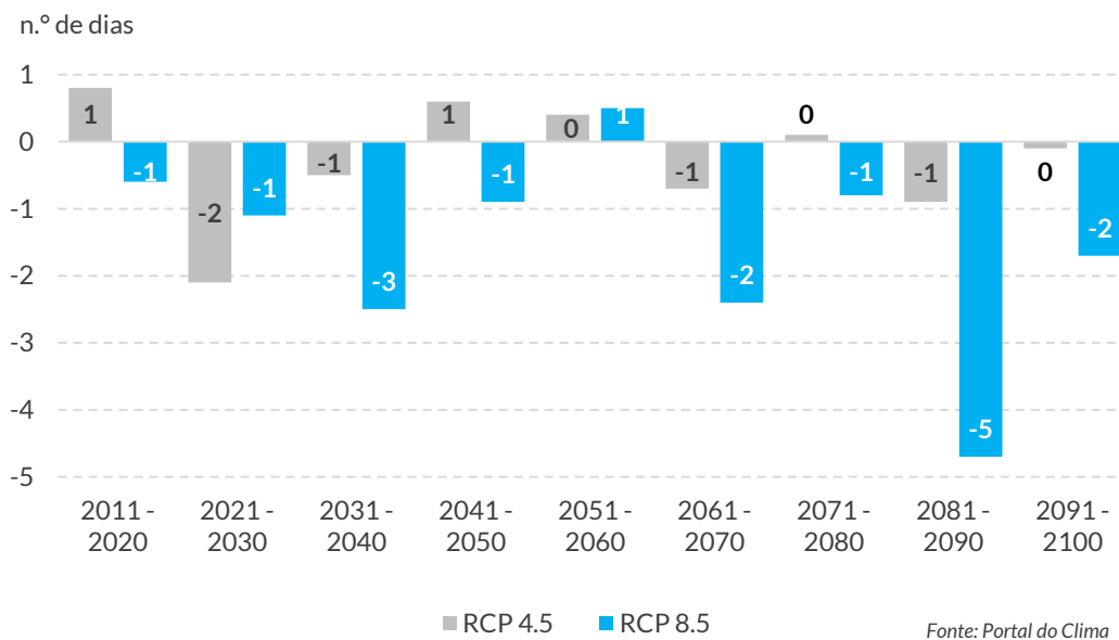
Gráfico 30. Anomalias de dias com precipitação superior a 20mm (n.º) na região de Viseu Dão Lafões
